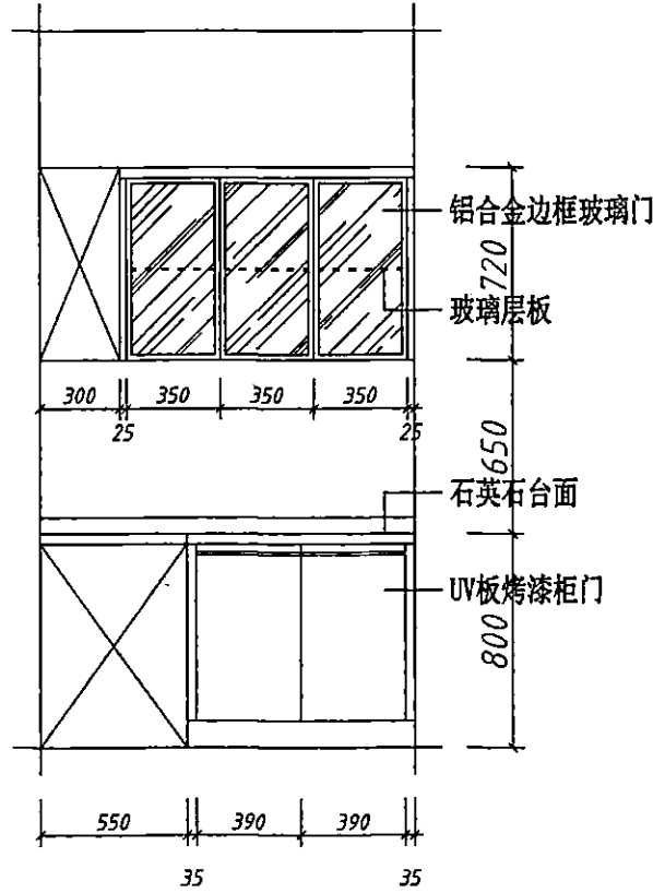
A立面大样图
