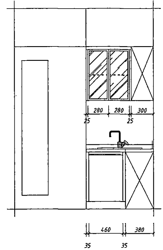
D立面大样图
